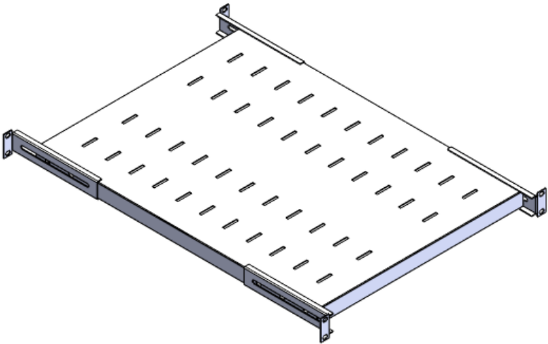
Изометрия
