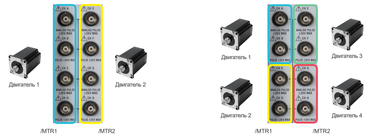
Один WT5000, сконфигурированный для одновременных синхронизированных измерений от 2 двигателей, для определения крутящего момента, скорости вращения, направления и электрических углов фаз A/B и Z Один WT5000, сконфигурированный для одновременных синхронизированных измерений с 4 датчиков крутящего момента и вращения, чтобы определить полный кпд 4 двигателей
