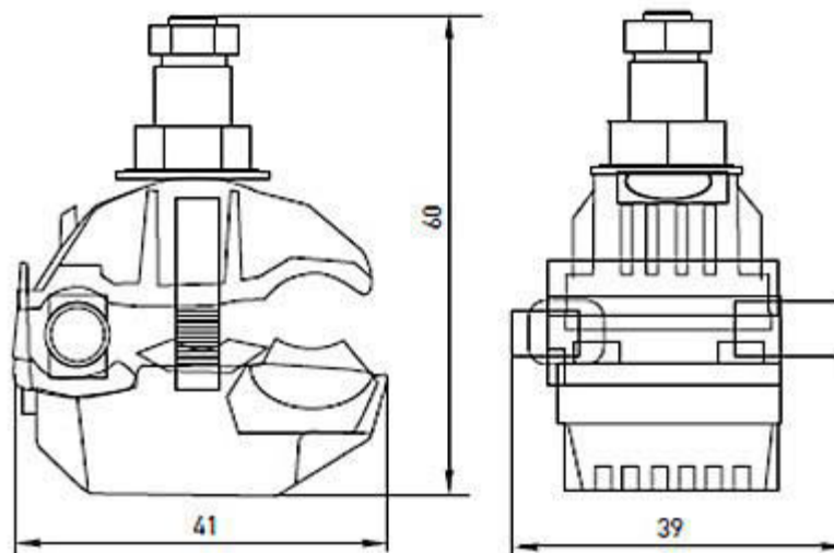
зажим прокалывающий ответвительный P1x-95
